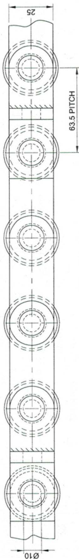
ELEVATION
